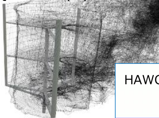
QBlade解析(例)
